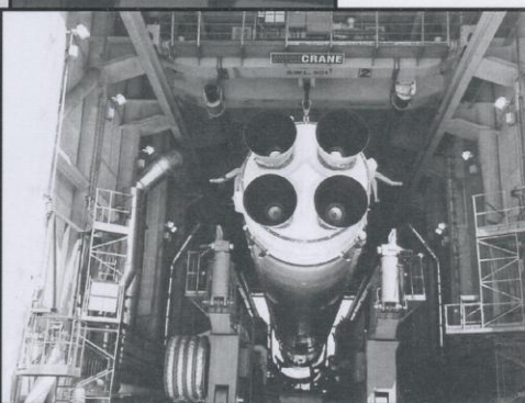
Over: Om trykken er rettferdig - vi ser en av 2 traverskraner fra Molde Cranes som er med på å transportere raketten fra dock til utskytingsposisjon. Stålprodukter AS er på plass - der kvalitet teller!
